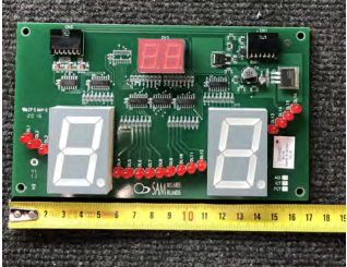
P. DISPLAY A.H. BABY 1.5” REF. 12229
